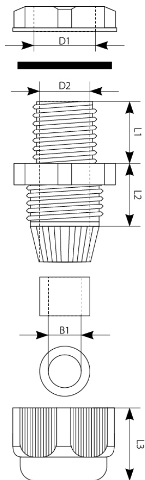
Rysunek Techniczny - Dławnica PG-13,5 IP68
