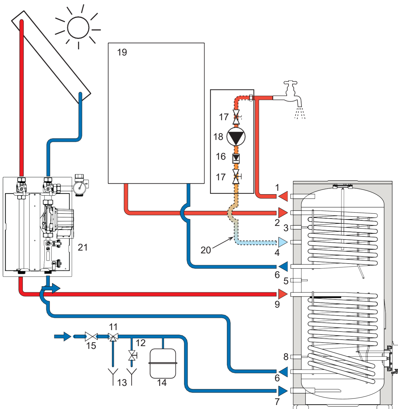
Rys. 6 – Układ hydrauliczny ECOUNTIT F 2C
