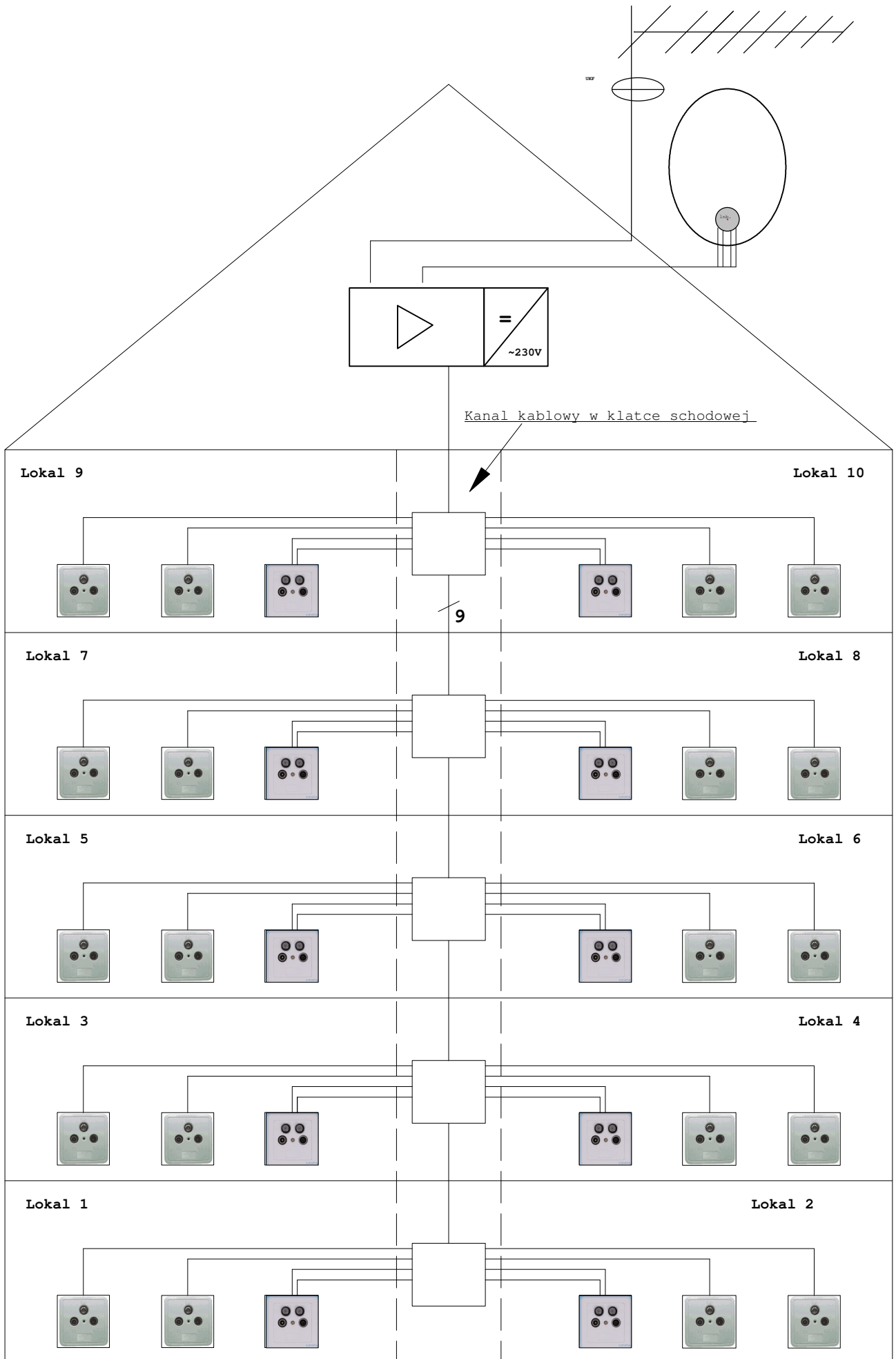
Przykładowa instalacja TV - SAT , budynek wielorodzinny
